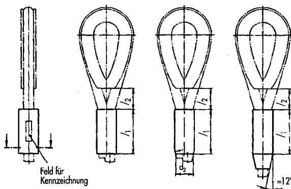
Pressklemme nach DIN 3093-2 mit Schlaufe und Kausche
