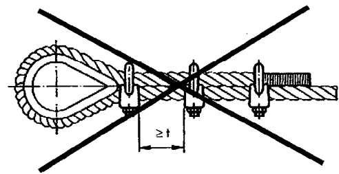
Drahtseilklemme nach DIN 1142 (nicht zulässig!)
